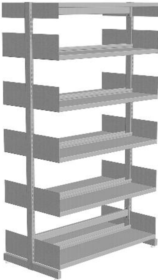
Ausführung mit rechteckigen Konsolen
