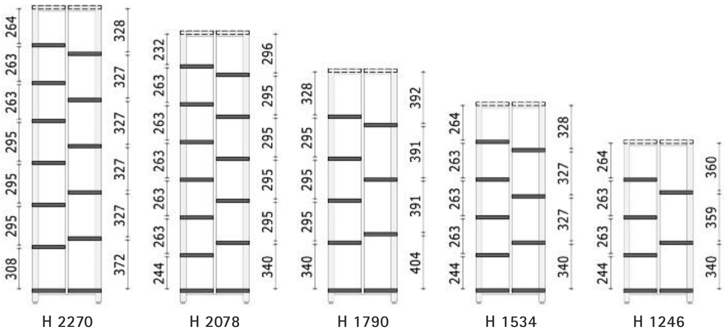
Regal-Höhenmaße für die Regalsysteme R.1–R.6 (inkl. Bodenausgleichsschraube)/Fachbodenaufteilung = Lichtmaß
